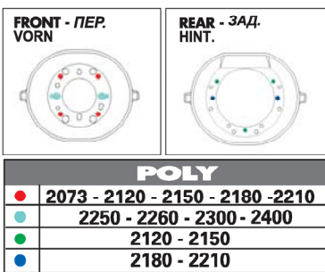
Plain safety cones - Защитные чехлы Schutzhauben
